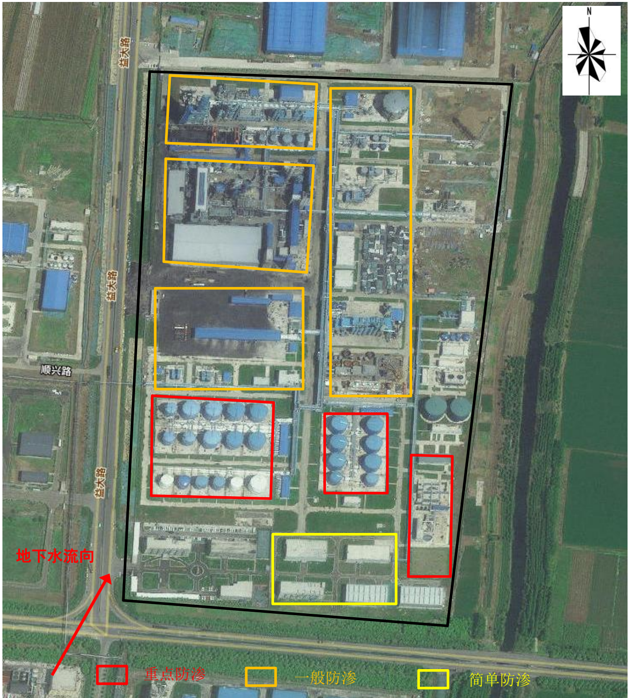
附图2 厂区分区防渗图
