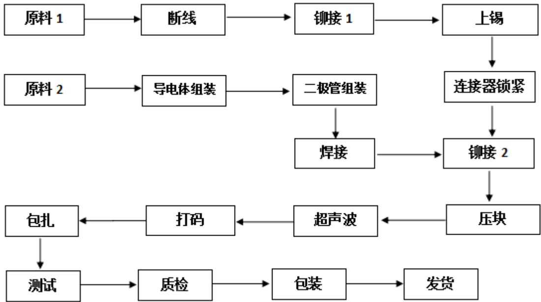
图 3 光伏接线盒生产工艺流程图
