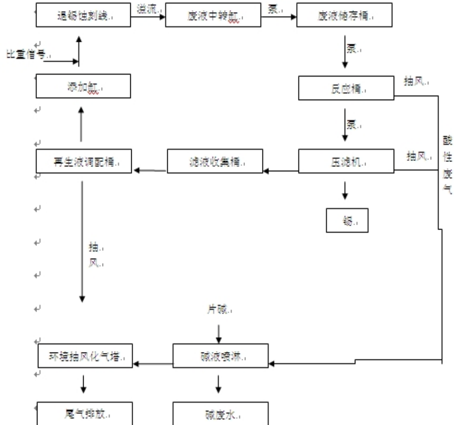
退锡废液循环再生处理系统工艺流程图
