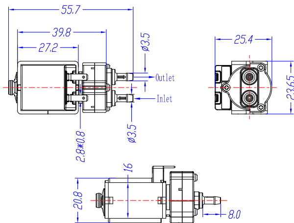
Dimensions/ 单位: millimeters/ 毫米
