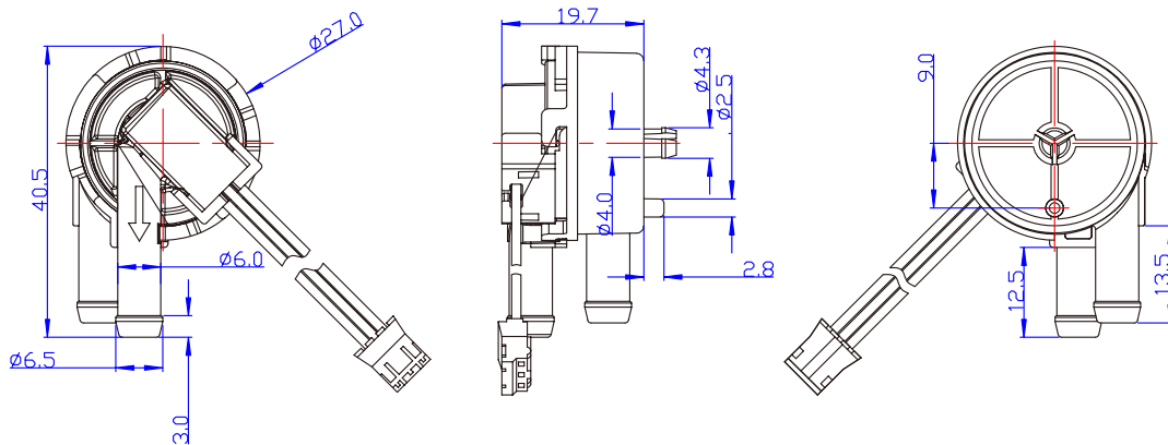
Dimensions/ 单位: millimeters/ 毫米
