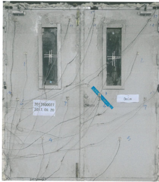
照片 1 耐火试验前试件情况
