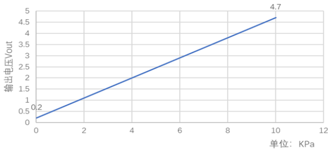
输出曲线 (以 10kPa 量程为例)
