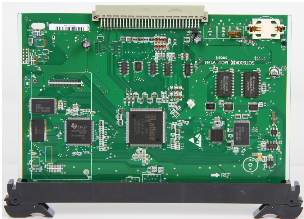
图 2-3 MCU 主控板
