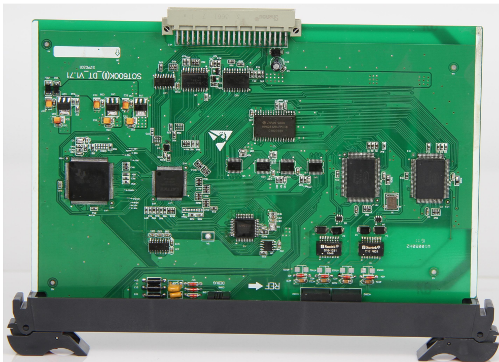
图 2-6 数字中继板
