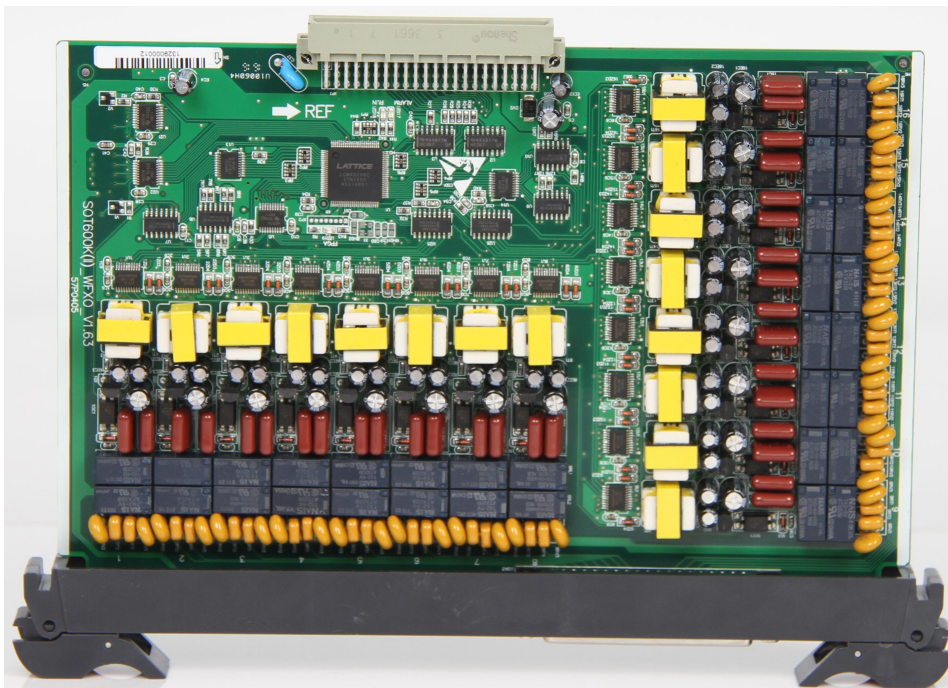
图 2-5 FXO 中继板
