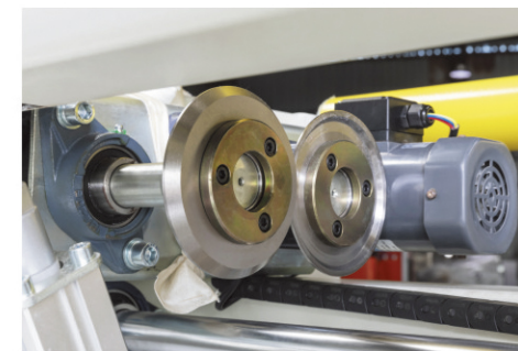
边刀 / Edge cutting
