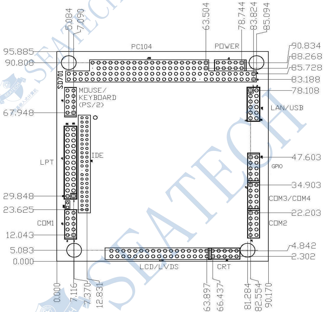
SD701 尺寸图 (单位: MM)
