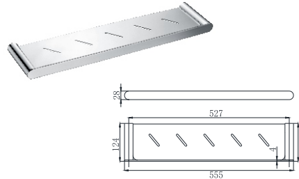
15-8809 Metal Shelf Chrome
