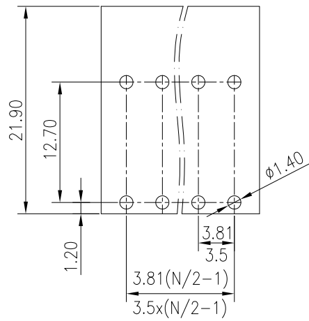
SECTION A-A P.C.B. LAYOUT
