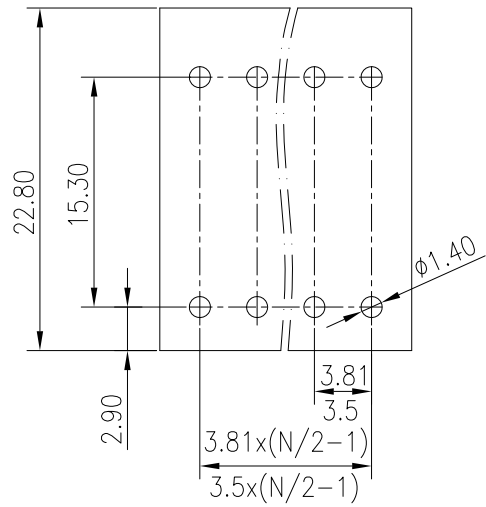
P.C.B. LAYOUT
