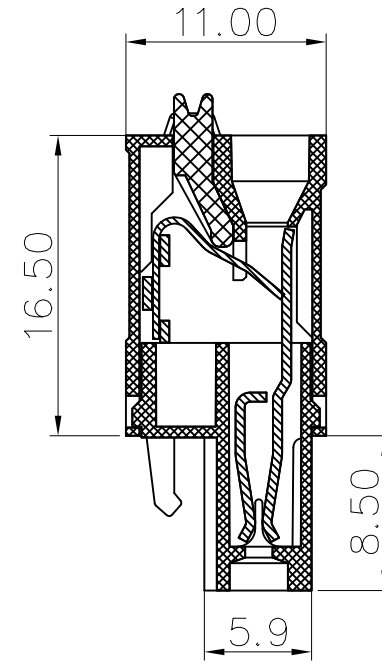
SEC A-A
