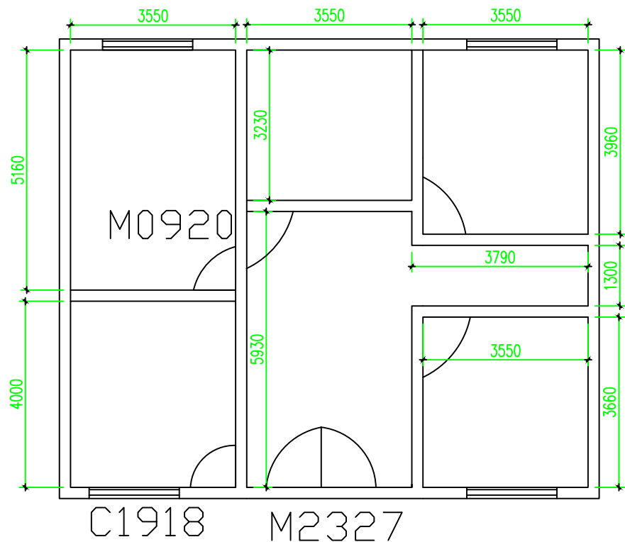
一层平面图
