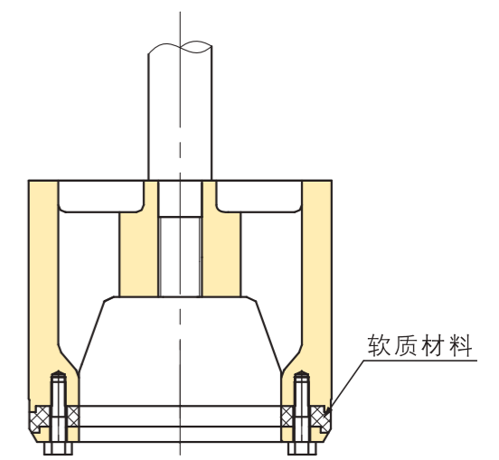
图6 切断型(Q型) 阀芯
