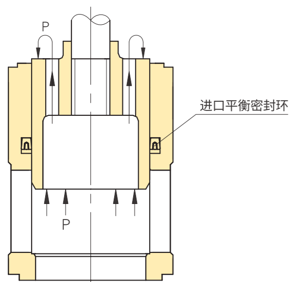
图2 平衡示意图
