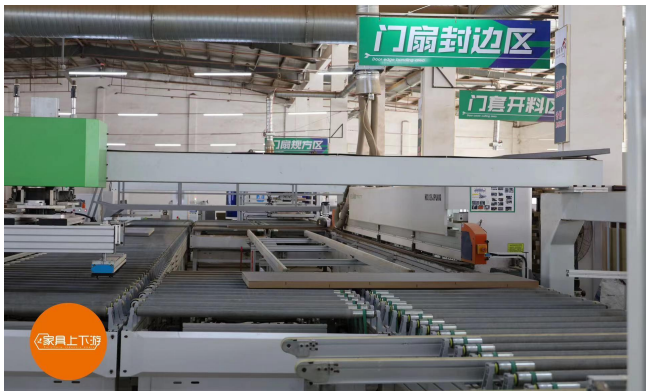
▲门扇封边区
