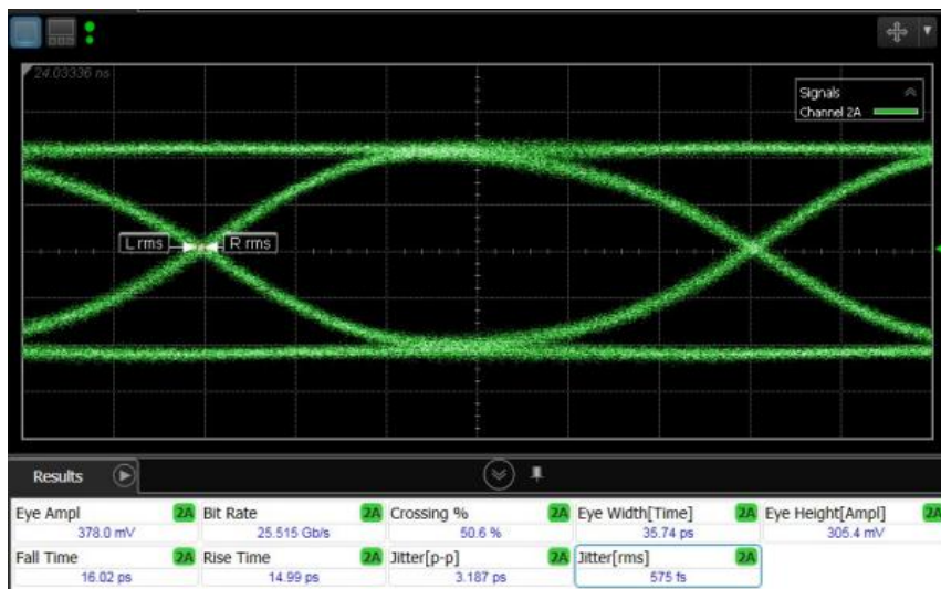
电眼图，测试条件：25.78G，PRBS31
