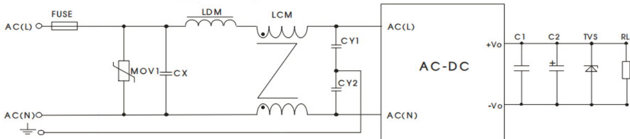
图2.EMC更高要求推荐电路
