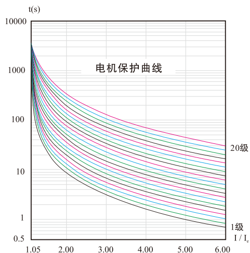
电机运行过程典型脱扣时间
