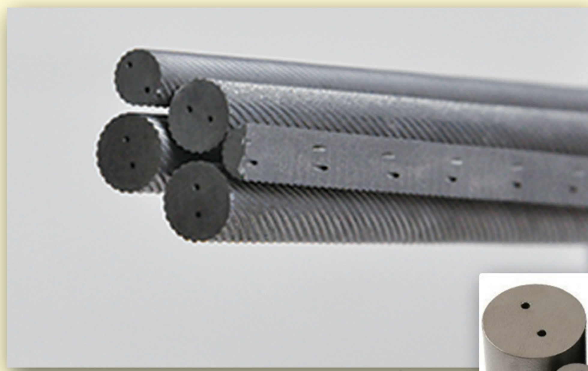
双螺旋孔圆棒材
