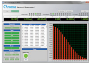
还原现场的失真波形
