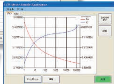
LCR标配软件所显示的扫频测量结果的明细图界面
